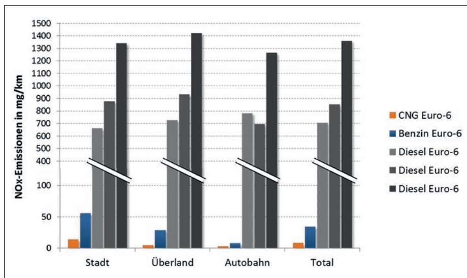
Abbildung 2: Auf der Strasse gemessene NOx-Emissionen von fünf Personenwagen mit verschiedenen Treibstoffen (CNG = Erdgas/Biogas), alle nach Euro-6b-Norm homologiert. Quelle: Empa
